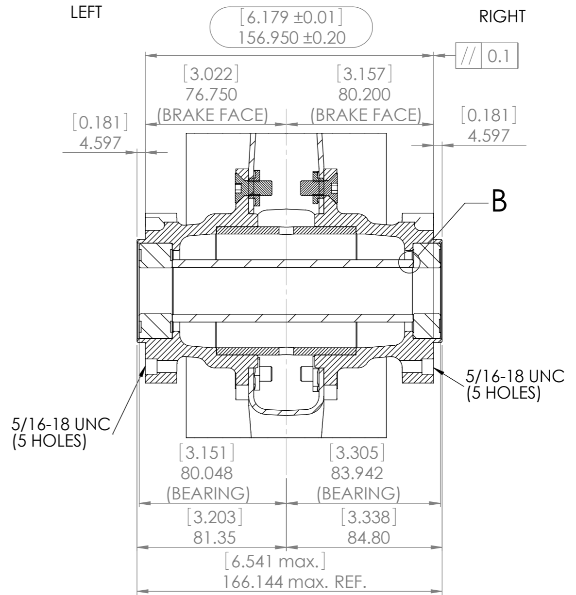
A-A (1 : 2)
