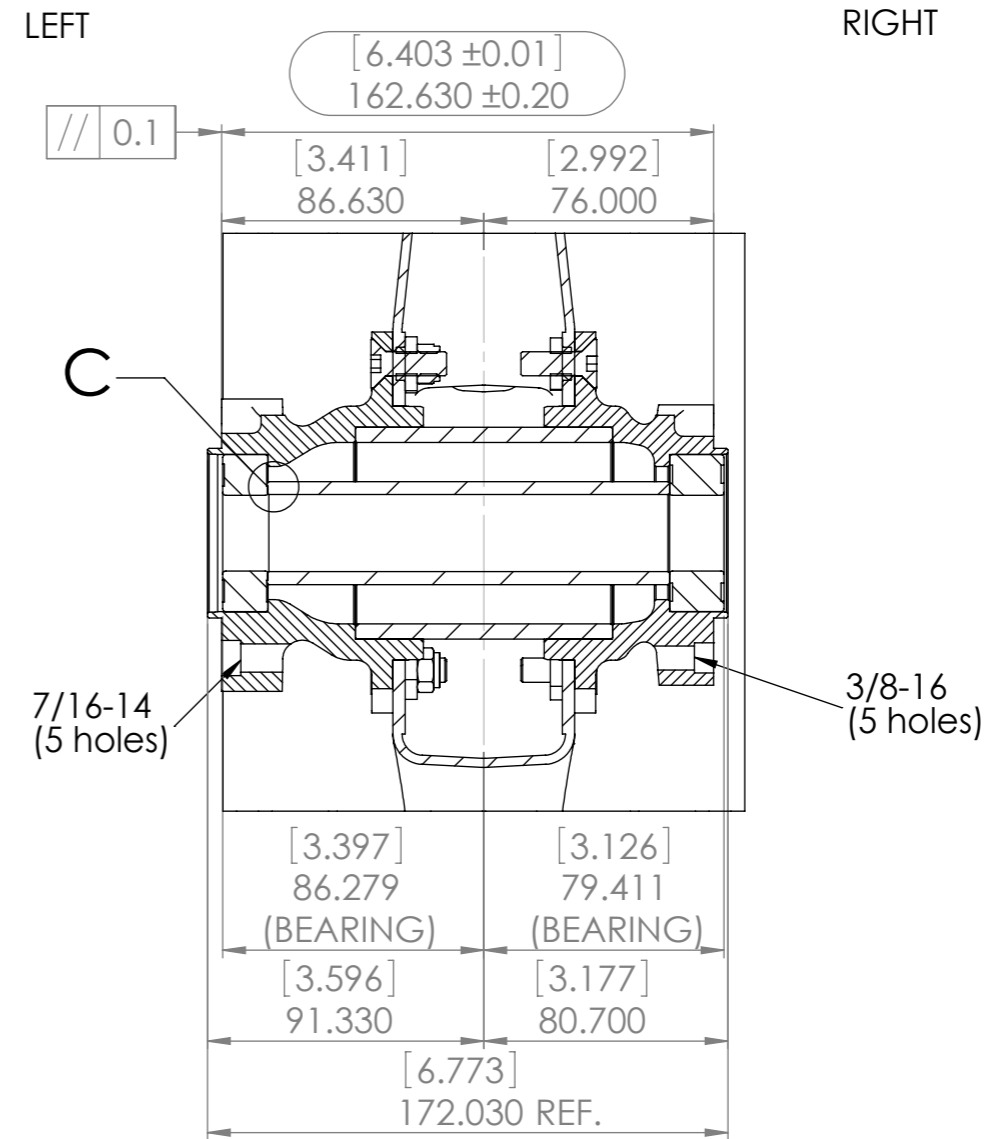
A-A (1 : 2.5)
