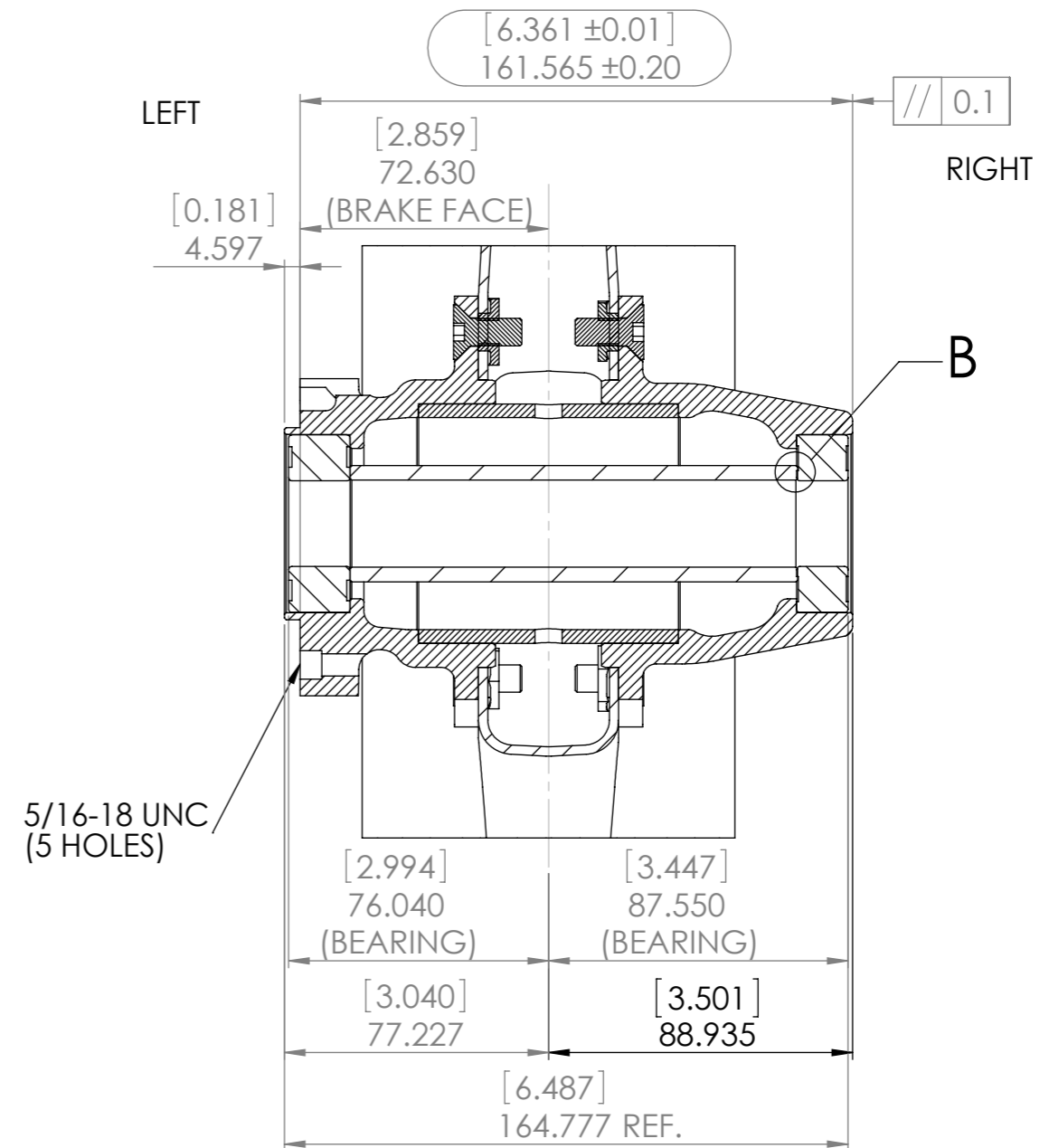
A-A (1 : 2)
