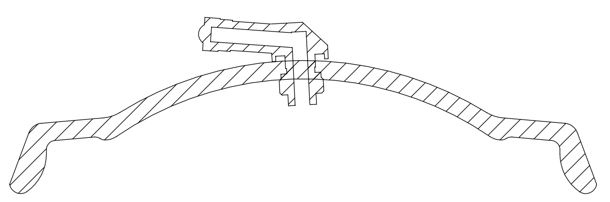
A-A (1 : 2)
