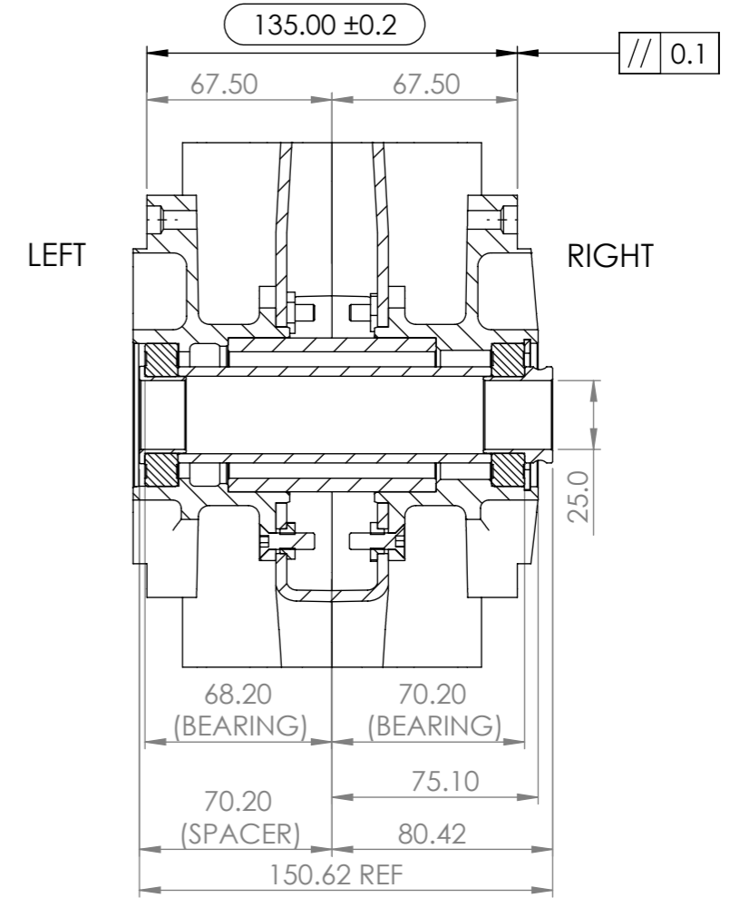
A-A (1 : 2.5)
