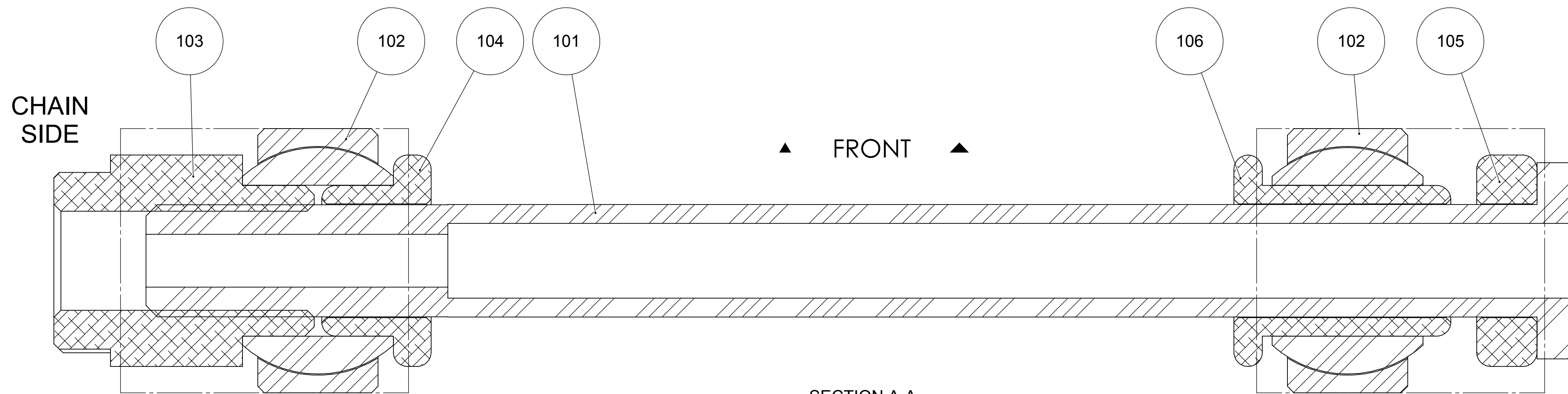
SECTION A-A
